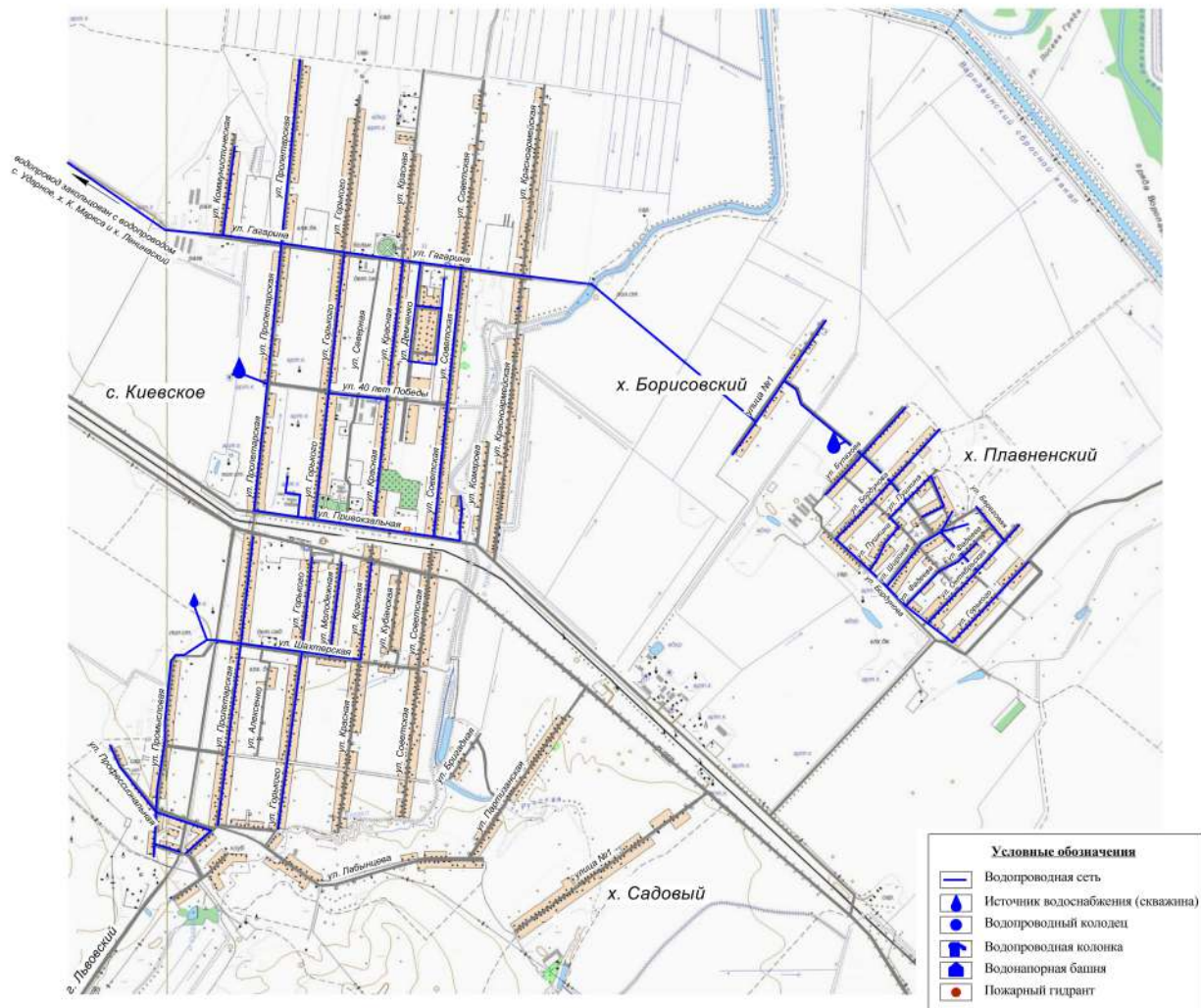
Рис. 1 - Схема водоснабжения с. Киевское, х. Борисовский, х. Плавенский
