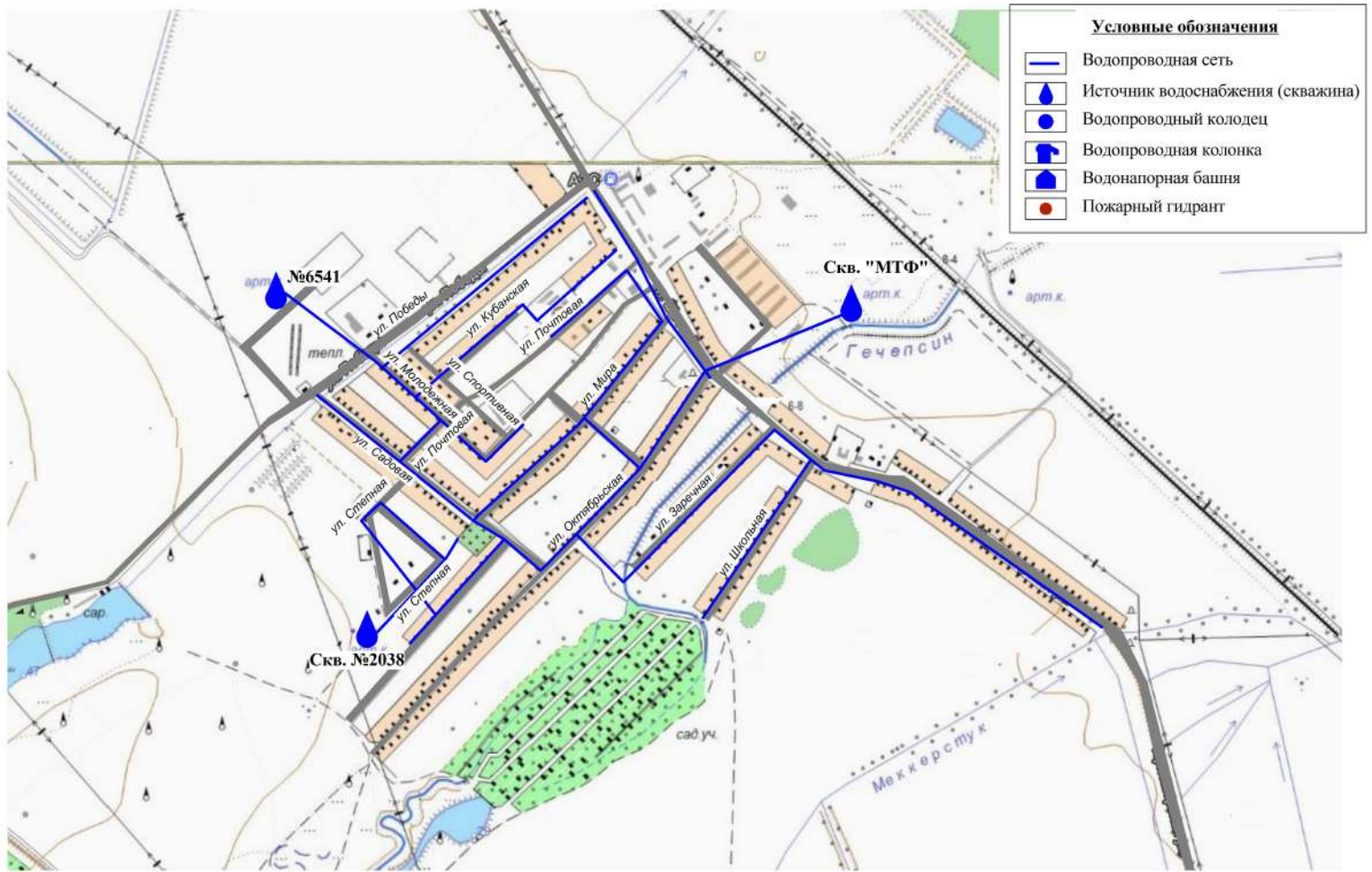
Рис. 3 - Схема водоснабжения с. Экономическое
