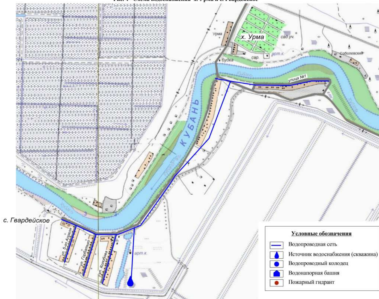
Рис. 4 - Схема водоснабжения х. Урма и с. Гвардейское
