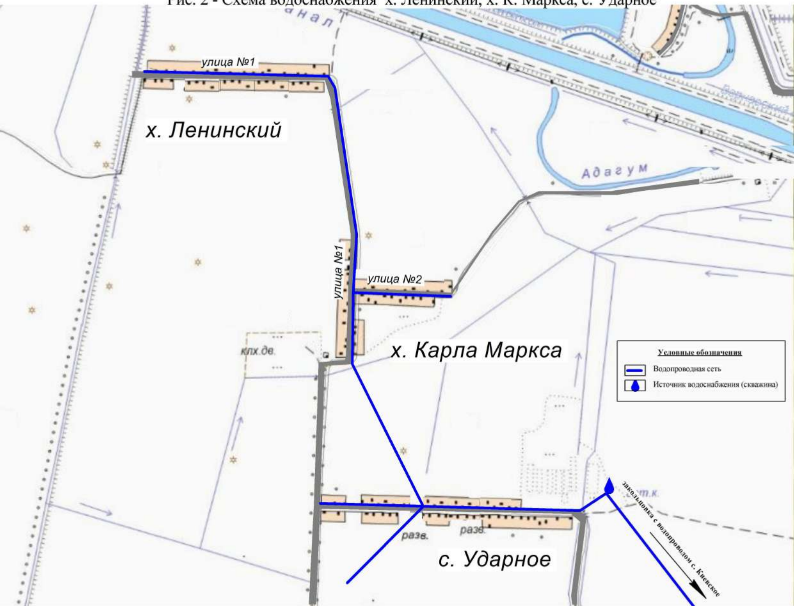
Рис. 2 - Схема водоснабжения х. Ленинский, х. К. Маркса, с. Ударное
